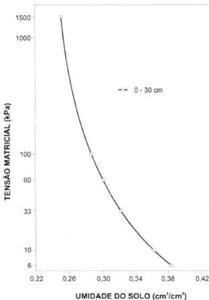
Figura 1 - Curva de retenção da água no solo.
