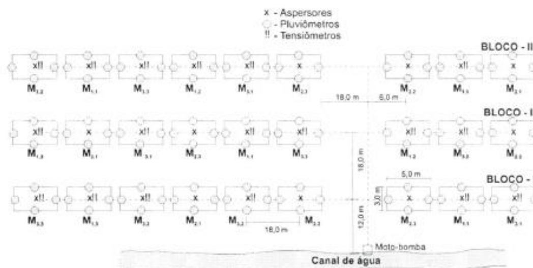
Figura 2 - Diagrama esquemático do ensaio.
