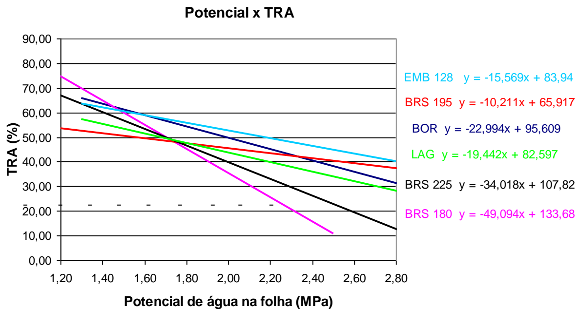
Figura 6. Representação gráfica do TRA x \Psi_f de seis cultivares de cevada - 2ª Avaliação.
